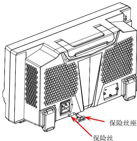
图 10 更换保险丝
