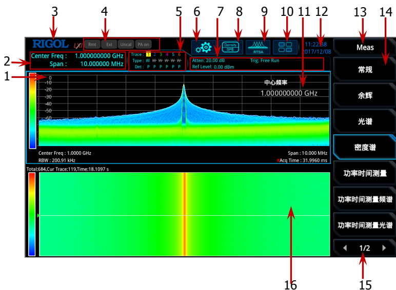
图 4 用户界面 (RTSA 模式)
