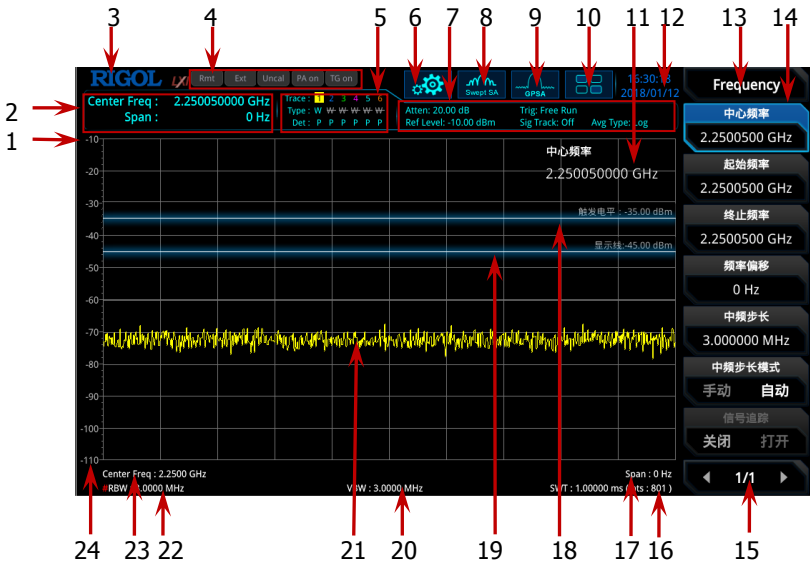
图 3 用户界面 (GPSA 模式)
