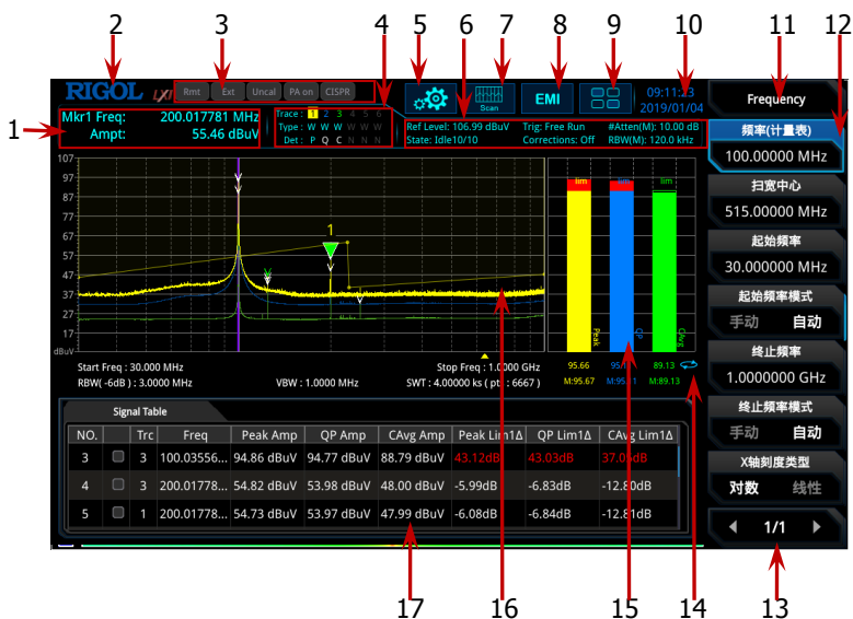
图 5 用户界面（EMI 模式）
