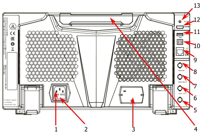
图 2 后面板
