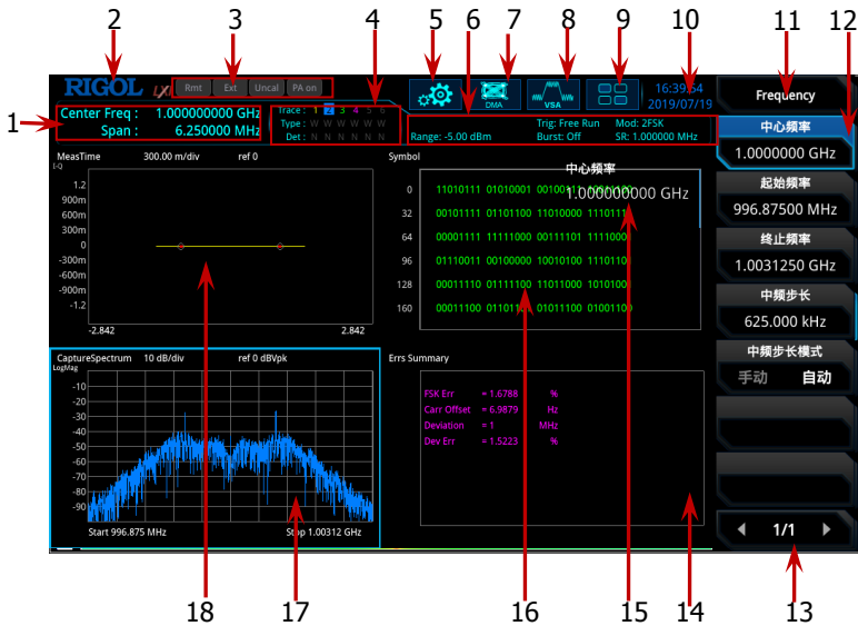
图 6 用户界面 (VSA 模式)
